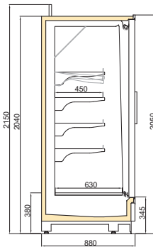
VINSON MT DGD/TKY 900/H2050
