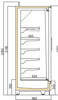
VINSON MT DGD/TKY 900/H2200
