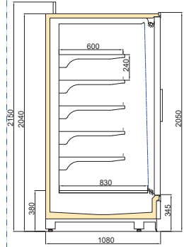
VINSON DGD/TKY 1100/H2050
