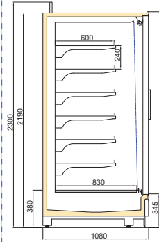
VINSON DGD/TKY 1100/H2200
