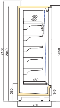
VINSON DGD/TKY 750/H2050
