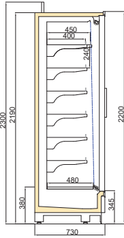
VINSON DGD/TKY 750/H2200
