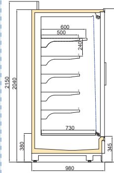
VINSON DGD/TKY 1000/H2050
