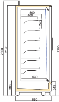
VINSON DGD/TKY 900/H2200
