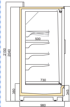
VINSON MT DGD/TKY 1000/H2050
