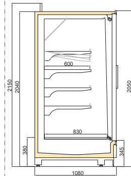
VINSON MT DGD/TKY 1100/H2050
