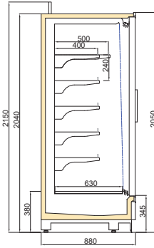
VINSON DGD/TKY 900/H2050
