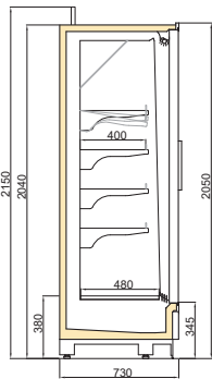
VINSON MT DGD/TKY 750/H2050
