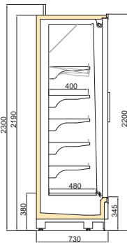
VINSON MT DGD/TKY 750/H2200
