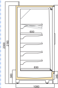
VINSON MT DGD/TKY 1100/H2200
