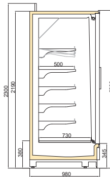
VINSON MT DGD/TKY 1000/H2200
