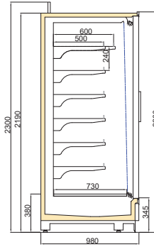
VINSON DGD/TKY 1000/H2200
