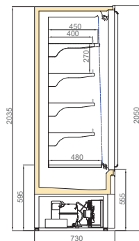
LISTER DGD/T55 750/H2050
