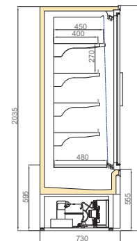
LISTER DGD/VNZ 750/H2050
