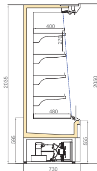
LISTER DP 750/H2050
