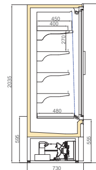
LISTER DGD/VWL 750/H2050
