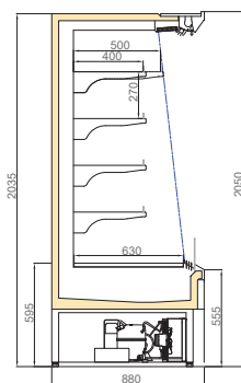
LISTER DP 900/H2050
