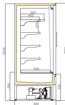
LISTER DGD/TKY 900/H2050
